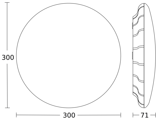
Maßzeichnung 1
